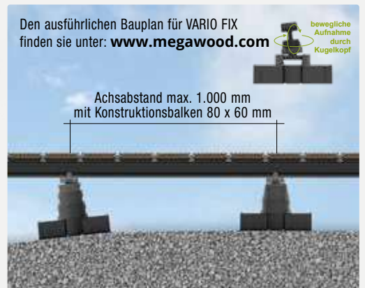
VARIO FIX II (44 - 242) Schwarz, 70 x 295 x 148 mm, mit Aufnahme für UK 40 x 60 mm und UK 80 x 60 mm
